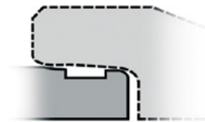
Giunto "CNZ" con sede tornita
