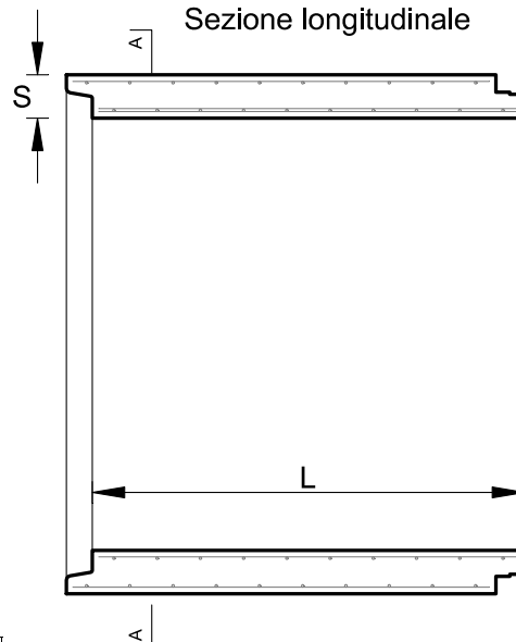
Sezione longitudinale
