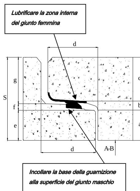
Particolare giunto
